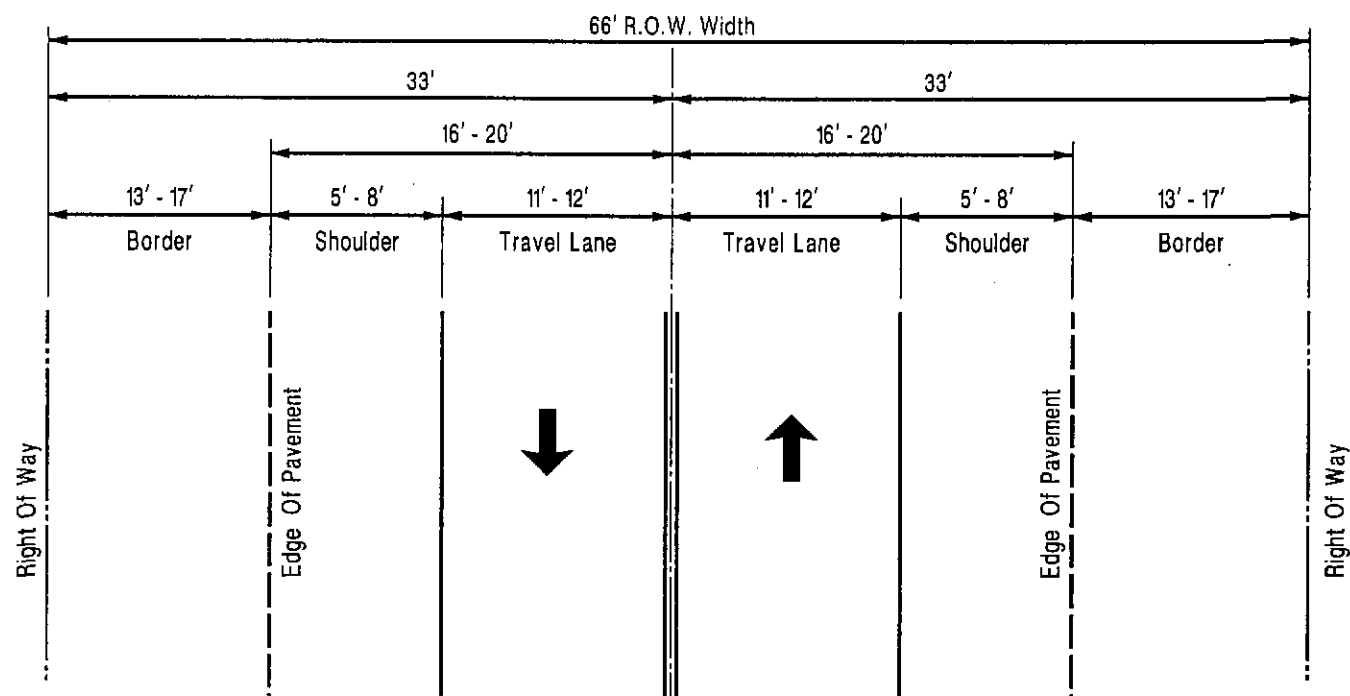
66' R.O.W. 2 LANE
