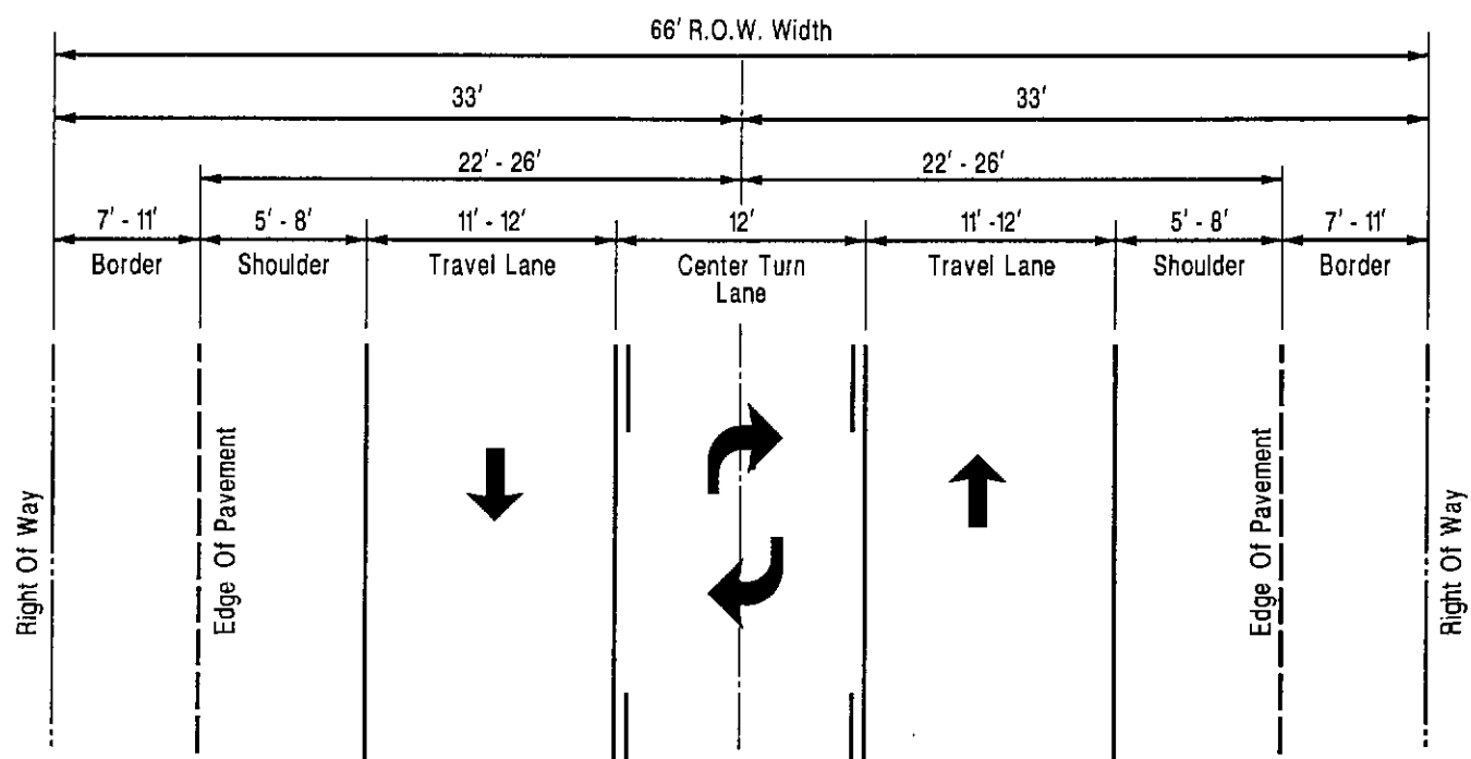
66' R.O.W. 3 LANE
