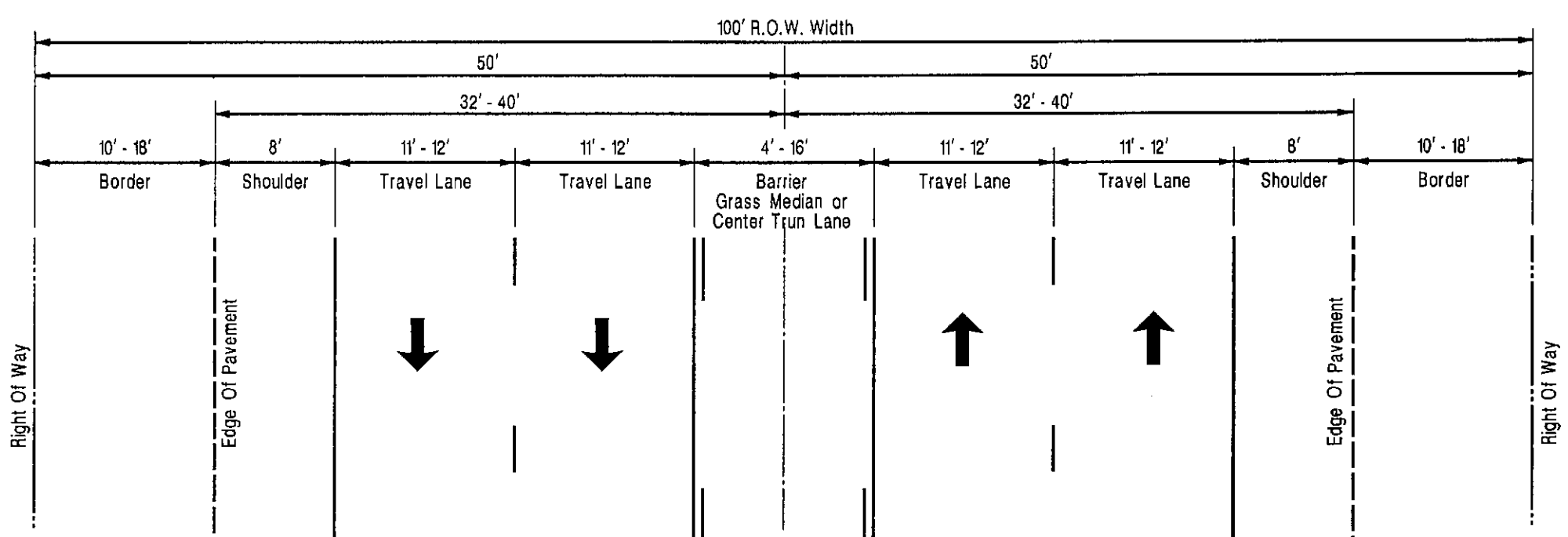
100' R.O.W. 5 LANE
